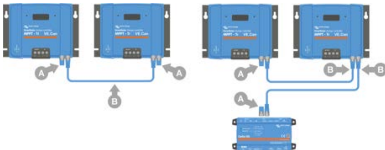
A: VE.Can-afsluiting - B: RJ45 UTP-kabel:
