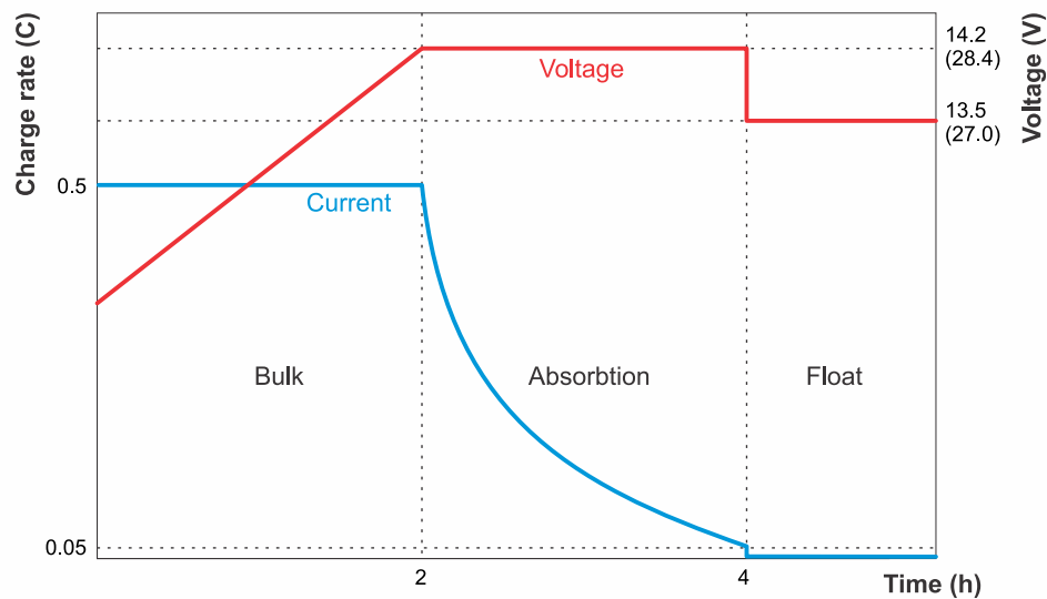
Lithiumacculaadgrafiek
